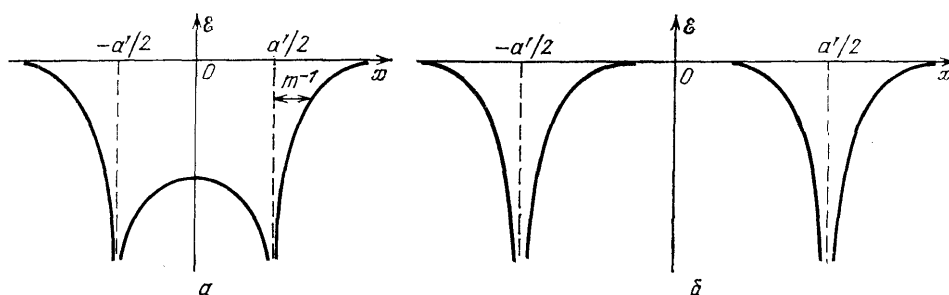
Рис. 2. Плотность вакуумной энергии (в вариантах a и b )
